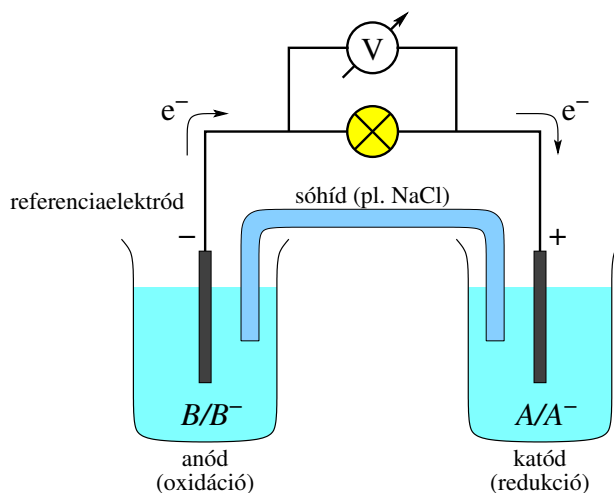
8.3. ábra. Elektrokémiai cella sematikus rajza.
