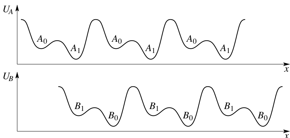
10.6. ábra. A „power stroke” racsní.
