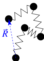
6.4. ábra. Kétdimenziós Gauss-lánc.
