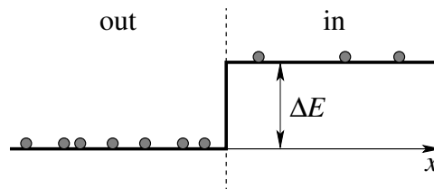
8.2. ábra. Két, membrán által elválasztott térrész, \Delta E energiakülönbséggel.
