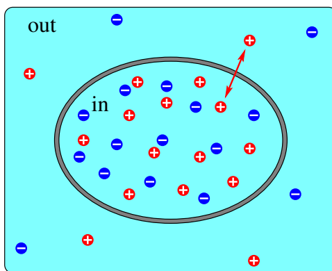
9.2. ábra. Az egyensúlyi Nernst-potenciál kialakulása.
