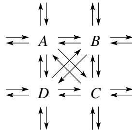
10.2. ábra. Többállapotú rendszer.
