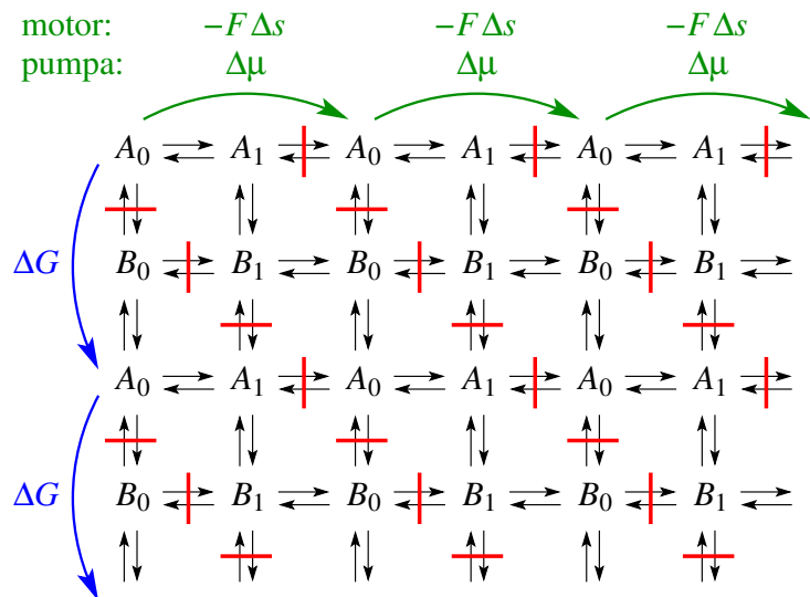
10.4. ábra. A kemomechanikai csatolás kétdimenziós rácsmodellje.
