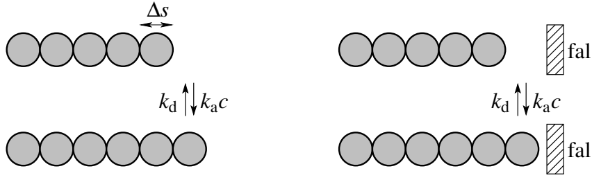
10.8. ábra. A polimerizáció egyszerű modellje.
