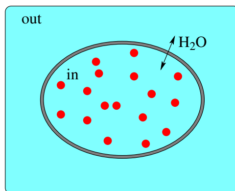
9.1. ábra. Az ozmózis jelensége.
