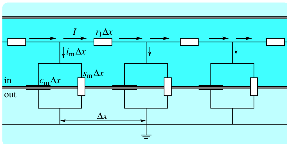
9.5. ábra. A passzív ingerületterjedés kábelmodellje, valamint a hosszanti irányban diszkretizált változatának helyettesítő áramköre.
