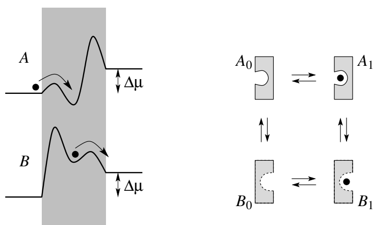
10.3. ábra. A molekuláris pumpák legegyszerűbb modellje.
