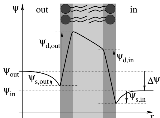
7.3. ábra. Az elektromos potenciál profilja egy membránon keresztül. A szaggatott vonallal ábrázolt szintek közötti nyilak talppontja a megfelelő potenciálkülönbség viszonyítási alapját jelzi.
