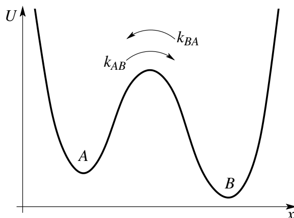
10.1. ábra. Kétállapotú rendszer energiatérképe a reakciókoordináta mentén.
