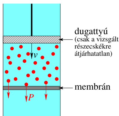
7.4. ábra. A permeabilitási együttható szemléltetése.
