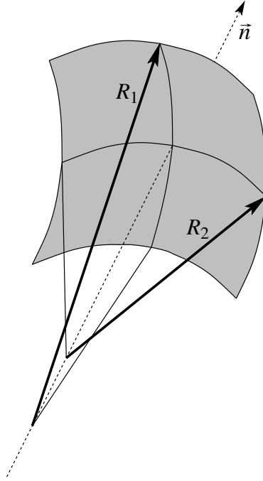
7.2. ábra. Egy görbült felület két főgörbületi sugarának ( R_1 és R_2 ) illusztrációja.
