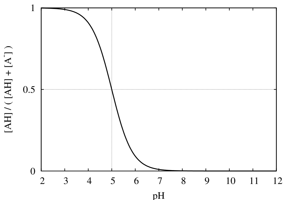
5.4. ábra. Példa titrálási görbére \text{p}K_a = 5 esetére.
