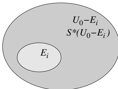
8.1. ábra. Kis részrendszer egy makroszkopikus rendszerben a Boltzmann-faktor illusztrációjára.
