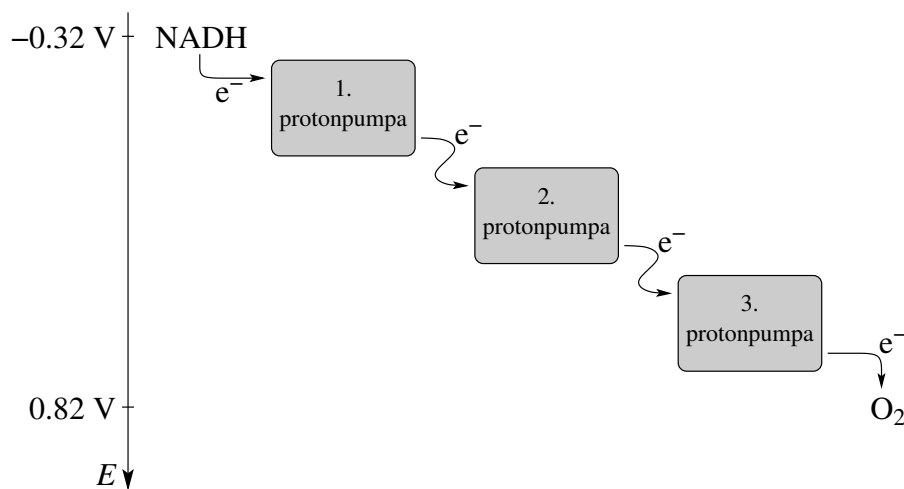
8.4. ábra. A NADH oxidációjához tartozó elektrontranszporlánc. A redoxpotenciál fentről lefelé nő.
