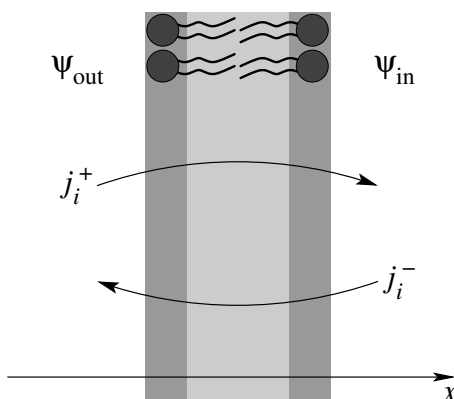
9.3. ábra. A membránon áthaladó ionok áramsűrűségei a külső és belső térrész irányából.
